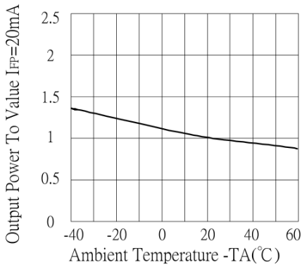
Intensity vs. Ambient Temperature Helligkeit über Umgebungstemperatur
