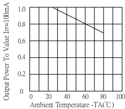
Intensity vs. Ambient Temperature Helligkeit über Umgebungstemperatur
