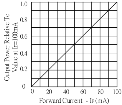
Radiant Intensity vs. Forward Current Strahlstärke über Flusstrom
