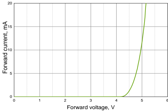
Forward Current vs. Forward Voltage Flusstrom über Flussspannung
